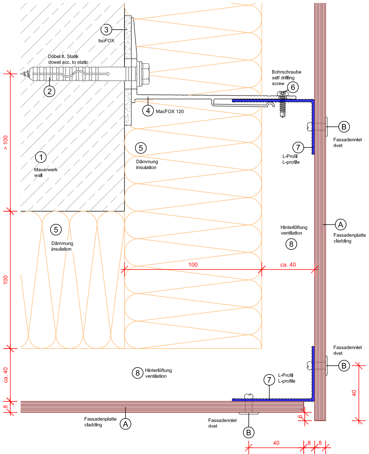
Horizontalschnitt - Aussenecke horizontal section - external corner
