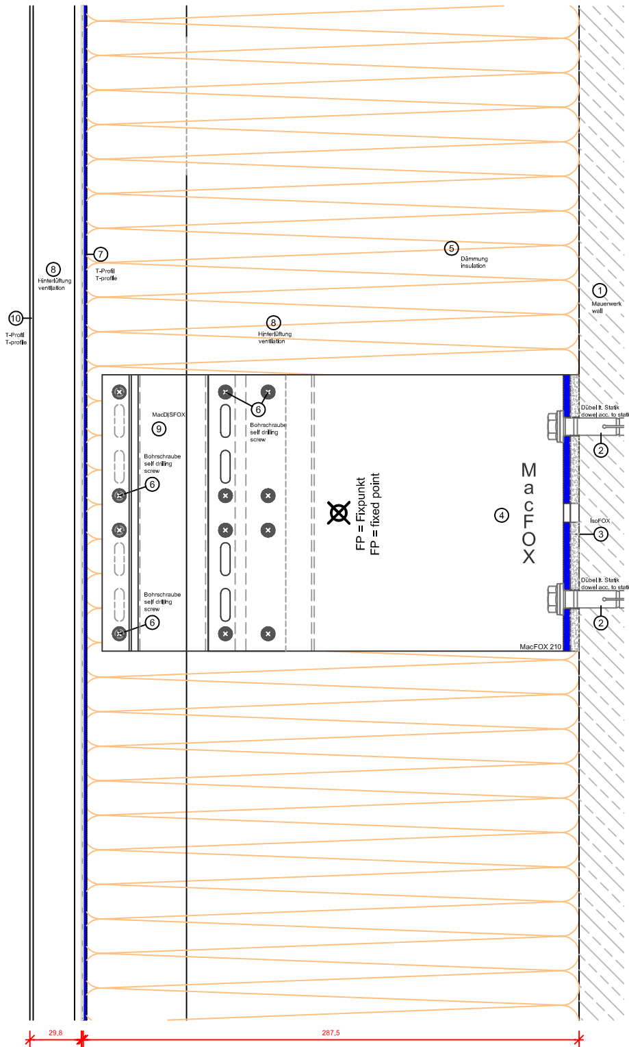
Vertikalschnitt - Haus der Wirtschaft vertical section
